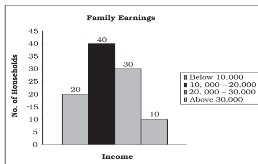
Fig. 8.3: Histogram
